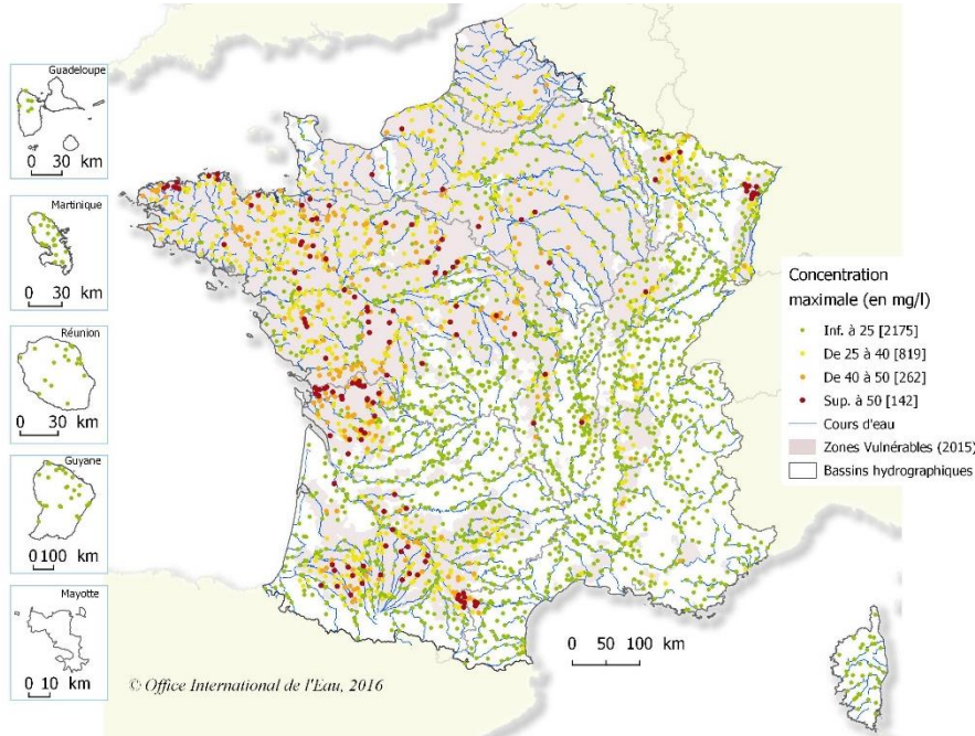
Figure 8 : Répartition spatiale des stations en eaux de surface selon les concentrations maximales en nitrates en 2014-2015
