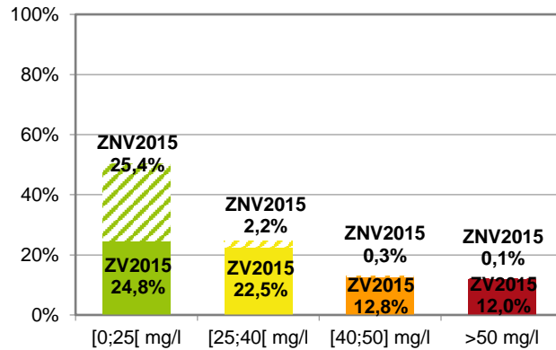
Figure 9 : Répartition des stations en eaux souterraines par classe de concentration moyenne en nitrates en 2014-2015
