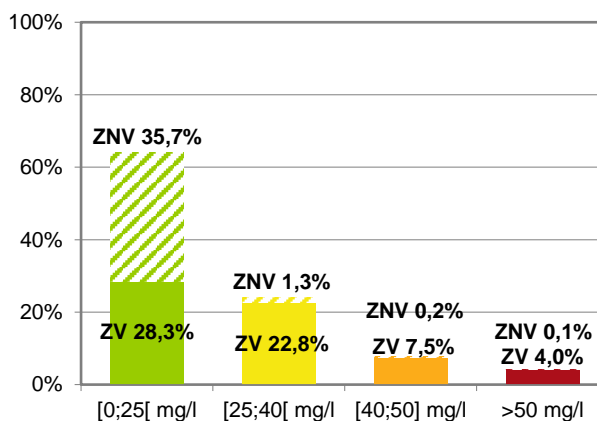
Figure 7 : Répartition des stations en eaux de surface par classe de concentration maximale en nitrates en 2014-2015
