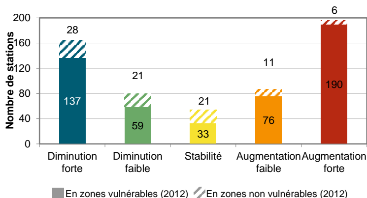
Figure 11 : Evolution des concentrations moyennes en nitrates des stations en eaux souterraines entre 1992-1993 et 2014-2015
