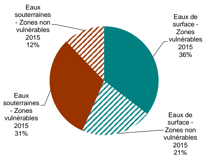
Figure 1 : Répartition des stations en 2014-2015 selon leur localisation en zones vulnérables (délimitation 2015)
