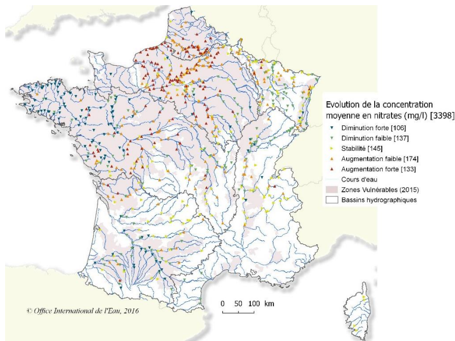
Figure 6 : Répartition spatiale des stations en eaux de surface selon l'évolution des concentrations moyennes en nitrates entre 1992-1993 et 2014-2015
