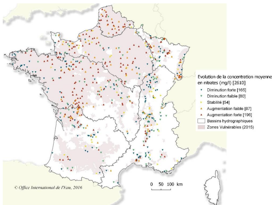
Figure 12 : Répartition spatiale des stations en eaux souterraines selon l'évolution des concentrations moyennes en nitrates entre 1992-1993 et 2014-2015
