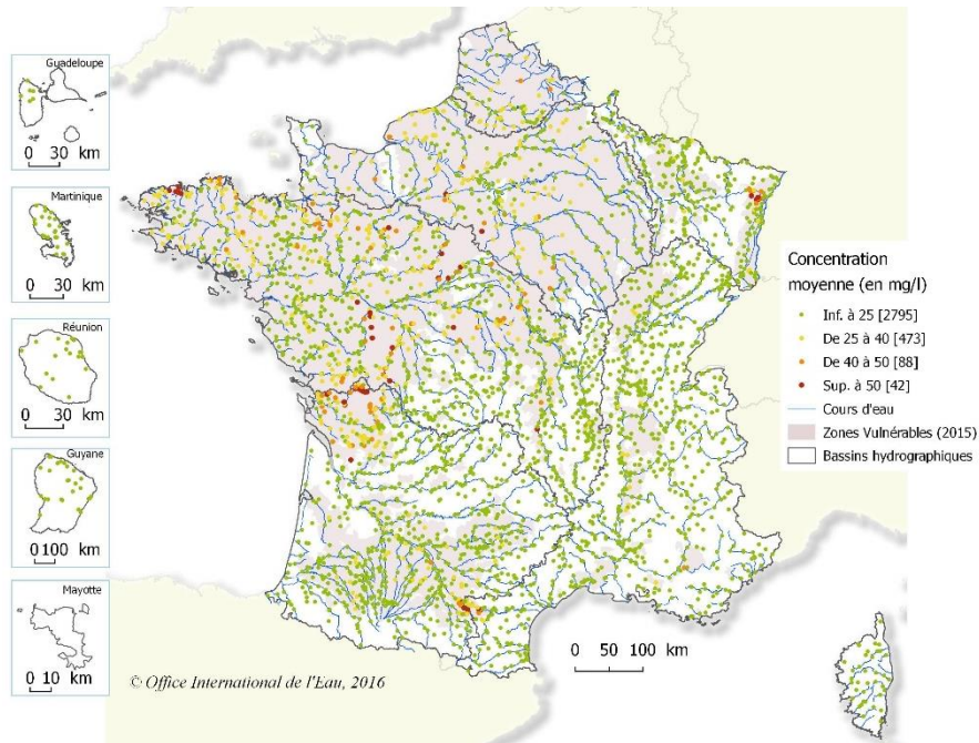
Figure 4 : Répartition spatiale des stations en eaux de surface selon les concentrations moyennes en nitrates en 2014-2015
