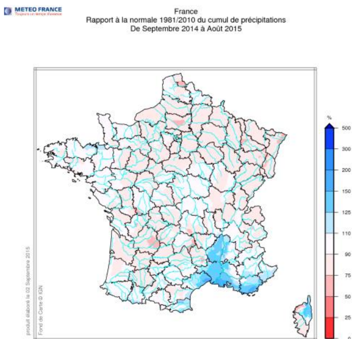
Figure 2 : Cumul des précipitations de septembre 2014 à août 2015
