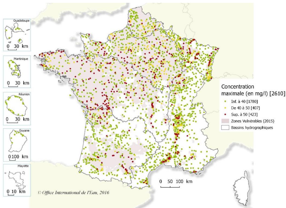
Figure 14 : Répartition spatiale des stations en eaux souterraines selon les concentrations maximales en nitrates en 2014-2015
