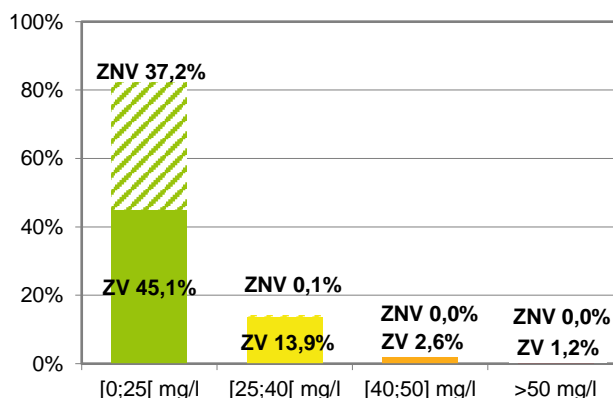
Figure 3 : Répartition des stations en eaux de surface par classe de concentration moyenne en nitrates en 2014-2015
