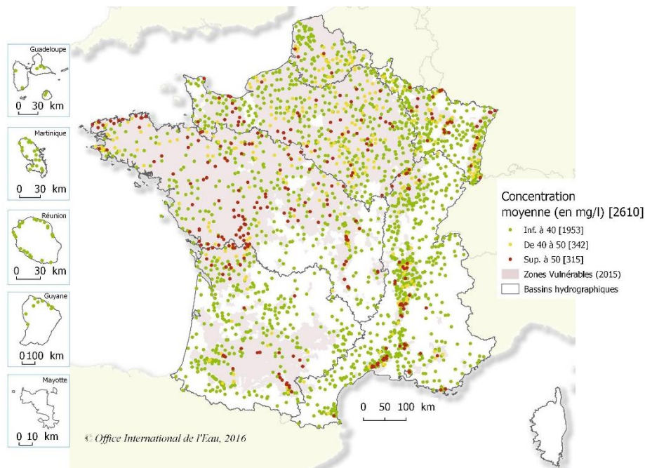
Figure 10 : Répartition spatiale des stations en eaux souterraines selon les concentrations moyennes en nitrates en 2014-2015
