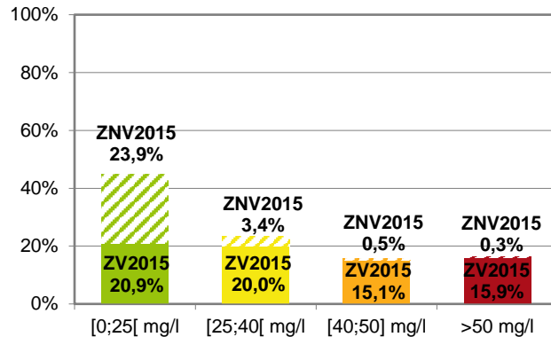
Figure 13 : Répartition des stations en eaux souterraines par classe de concentration maximale en nitrates en 2014-2015
