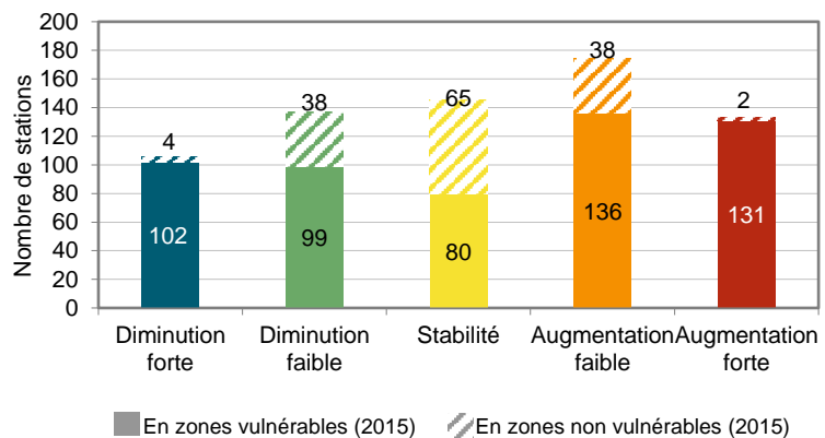
Figure 5 : Evolution des concentrations moyennes en nitrates des stations en eaux de surface entre 1992-1993 et 2014-2015
